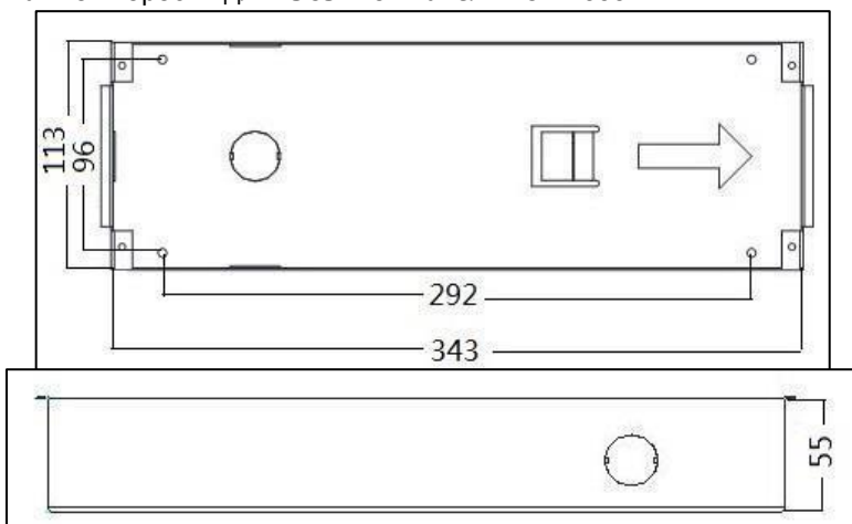
Рисунок 5-12 Вид спереди и сбоку
