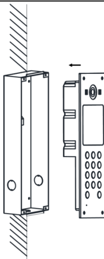
Рисунок 5-14 Установка вызывной панели 7.
