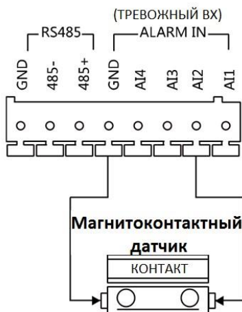
Рисунок 5-19 Подключение магнитоконтактного датчика для модели DSKD6002-VM
