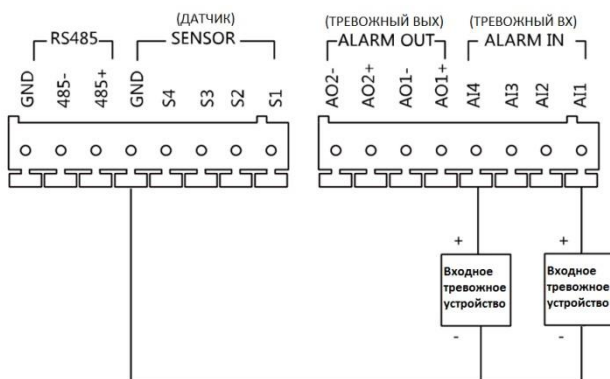
Рисунок 5-24 Подключение входов тревожных устройств для DS-KD8102-V/DSKD8002-VM
