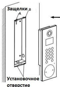
Рисунок 5-4 Установка вызывной панели
