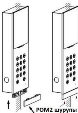
Рисунок 5-11 Закрепление вызывной панели
