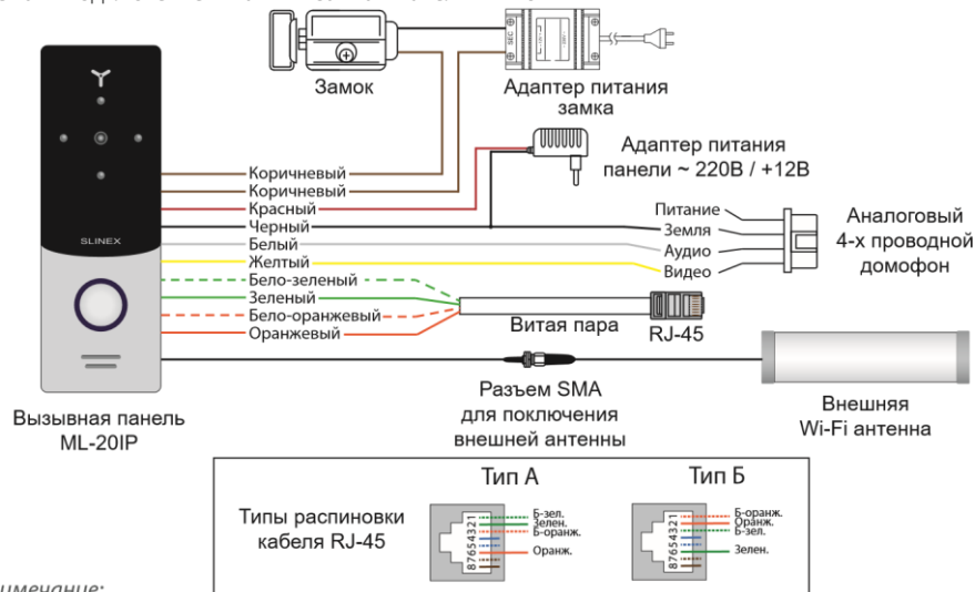
Схема 1. Подключение питания и замка к панели ML-20IP.
