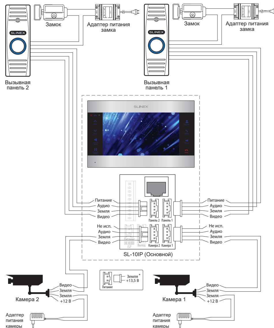
Схема 1. Подключение вызывных панелей и камер к домофону SL-10IP.
