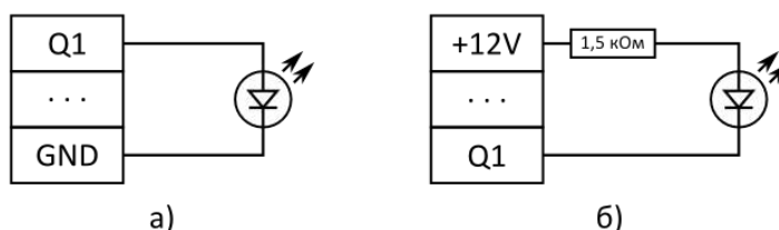
Рисунок 2.5 – Схеми підключення індикаторів підтвердження
