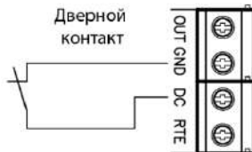
Рис.6. Подключение дверного контакта
