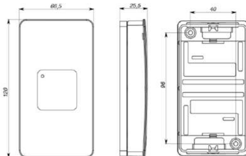
Рис 2. Габаритные размеры
