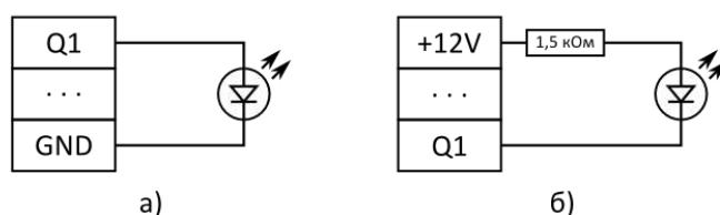
Рисунок 2.6 – Схеми підключення індикаторів підтвердження
