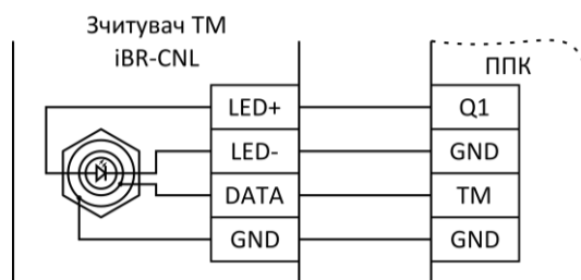
Рисунок 2.7 – Схема підключення зчитувача ключів TM
