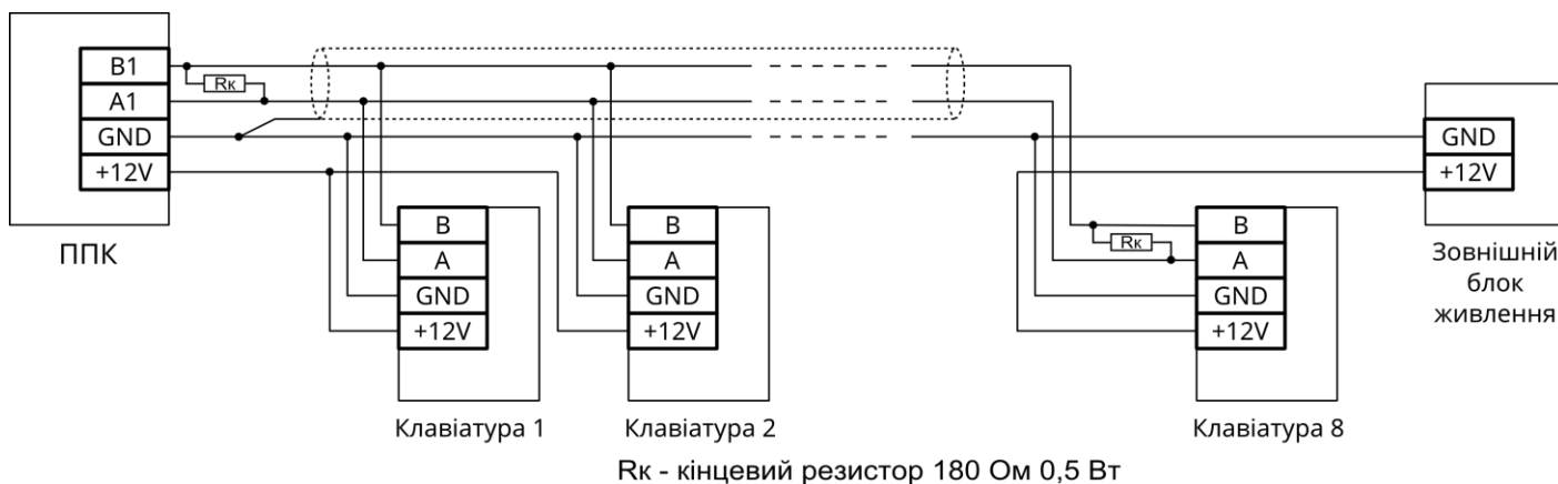
Рисунок 2.2 – Приклад підключення клавіатур по шині RS-485
