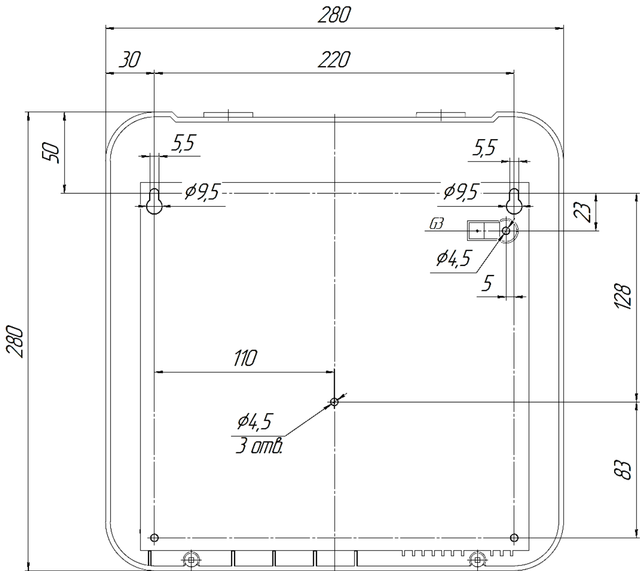
Рисунок 1 – Установчі розміри модуля M-ZP mBox
