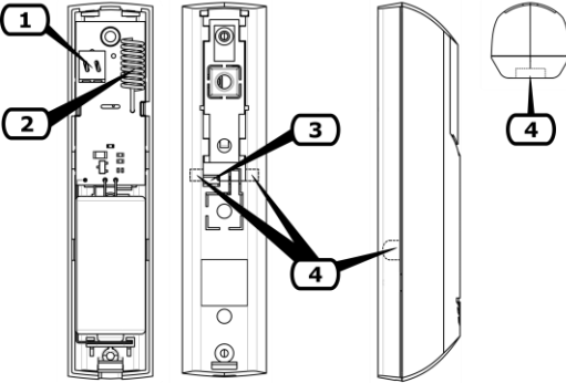
Рисунок 3.1 – Розміщення клемного з'єднувача, місць для прокладання дротів та вирізів 1 – Клемний з'єднувач, 2 – Антена, 3 – Місце для прокладання дроту, 4 – Місця для вирізів
