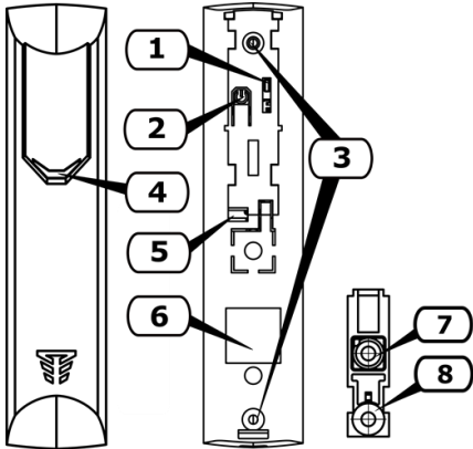
Рисунок 3.4 - Зовнішній вигляд елементів сповіщувача
