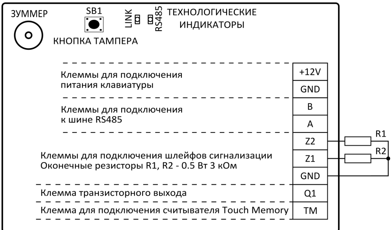
Рисунок 2 - Схема электрическая подключения
