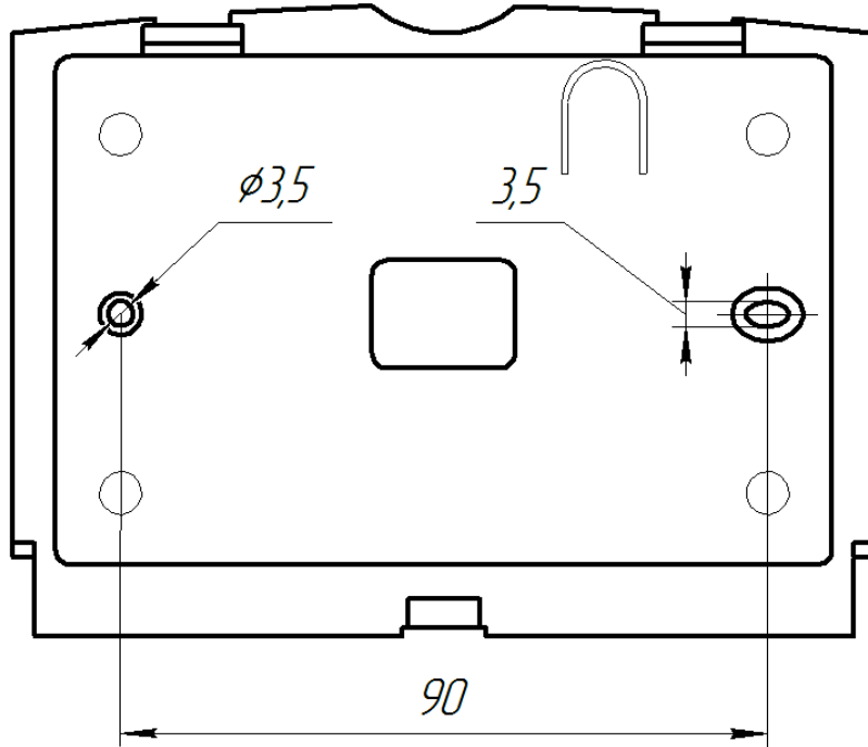
Рисунок 1 - Установочные размеры клавиатуры K-LED16
