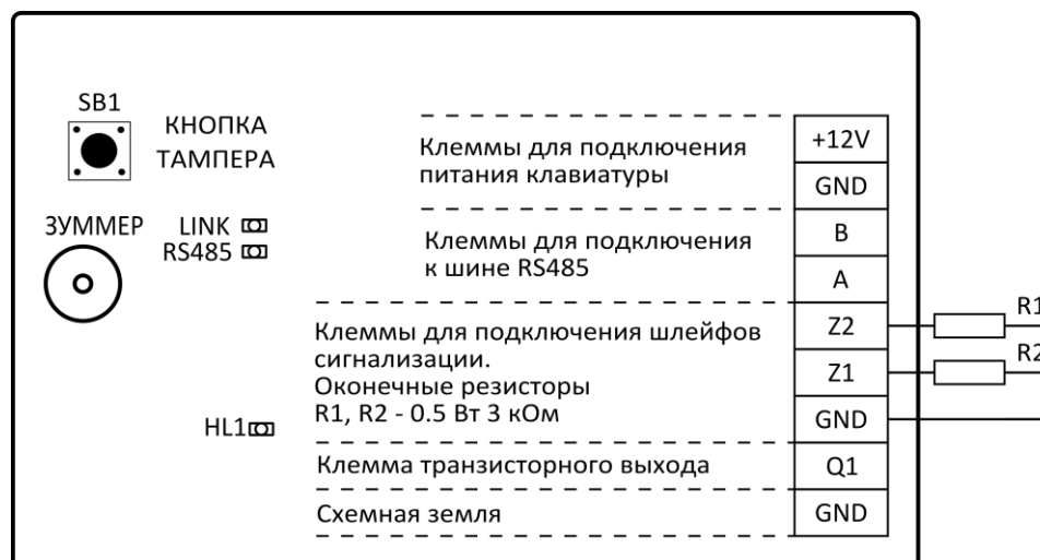
Рисунок 2 - Схема электрическая подключения
