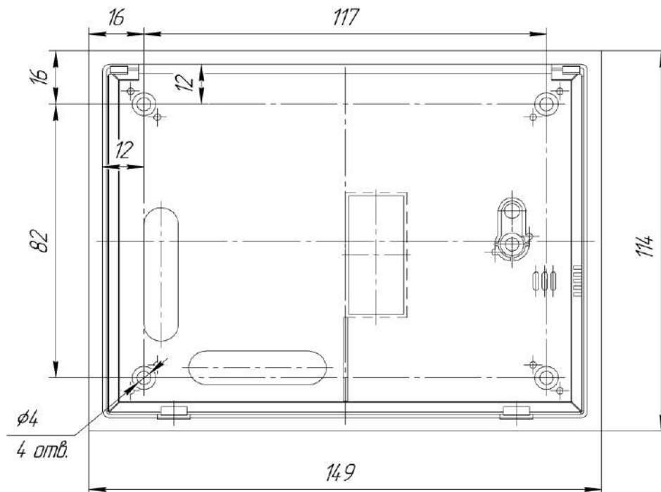
Рисунок 1 – Установочные размеры клавиатуры K-GLCD
