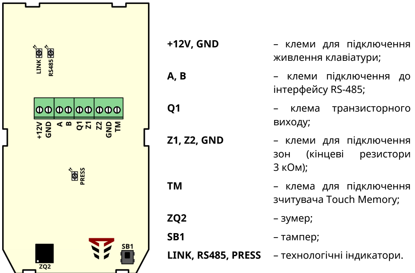
Рисунок 2 - Зовнішній вигляд та опис елементів плати клавіатури
